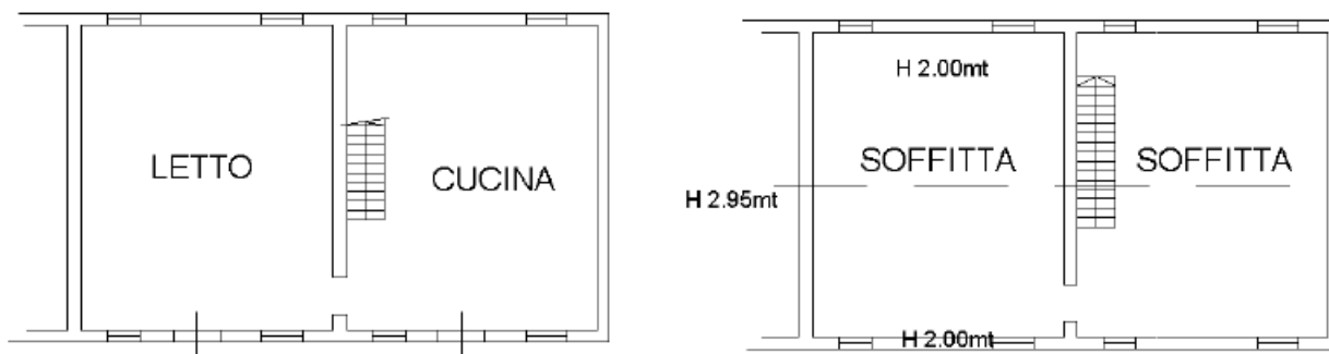
Pianta abitazione (piano terra – sx e piano primo – dx) – fuori scala -
