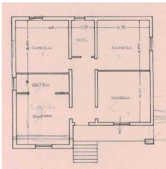
Pianta da Licenza edilizia
